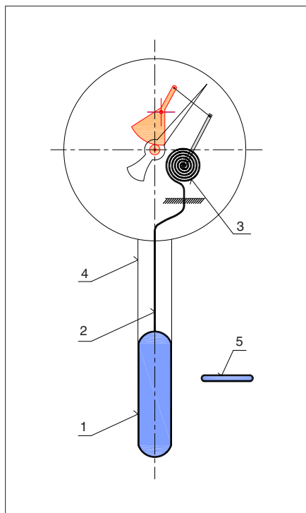
Obr. 1. Schéma plynového teploměru: 1 – plynové tělísko, 2 – kapilára, 3 – tlakoměrný deformační člen, 4 – stonk, 5 – průřez trubice, z níž je zhotoven deformační člen
