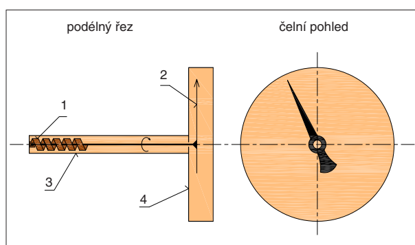
Obr. 3. Funkční schéma bimetalového teploměru: 1 – bimetalový deformační člen, 2 – ručka, 3 – stonk, 4 – tělo ukazatele a ciferník
